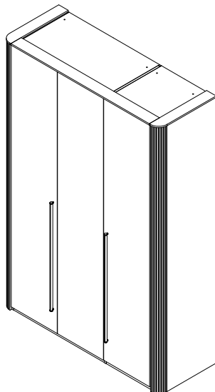
P3-10G/RO LWH - 1530X559X2248
