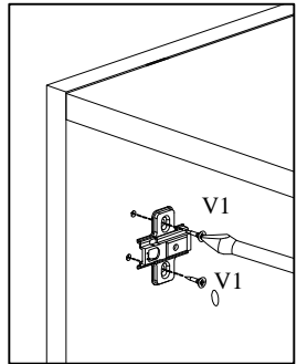
A DETAYI
