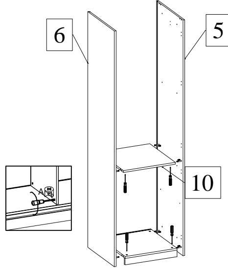
A DETAYI
