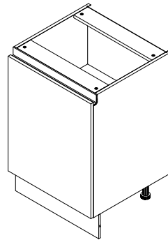
R-60-1K LHW-600X943X600
